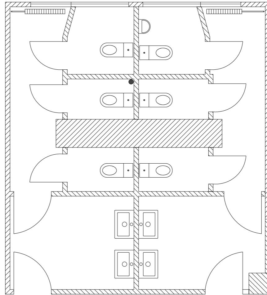
Parter projekt
