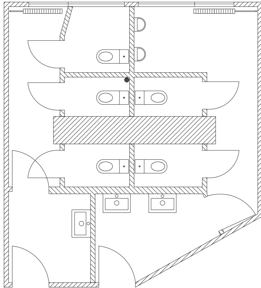
Parter inwentaryzacja
